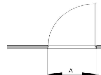
מידת רוחב פתח נקי בלוק לבלוק משקוף עיזור למשקוף עיזור (A)
